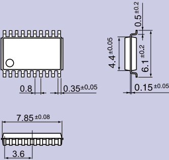
SSOP-20
